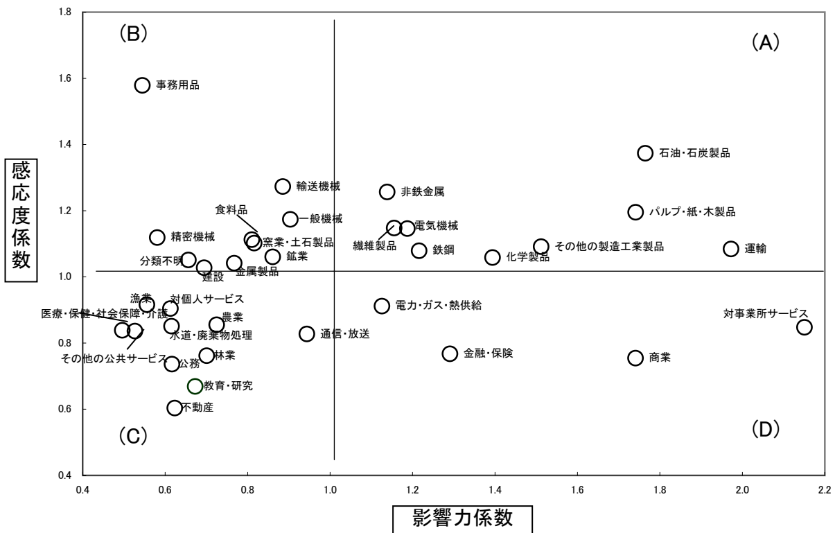
図 I -13 影響力係数と感応度係数(新鳥取市)
